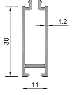
Profil No : KC0352 ⚠ Ağırlık : 274 gr/m ⚠ İşaretili profil için satış ekibinden bilgi alınız.
